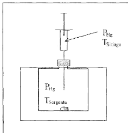
Figura 3 - Schema dell'unità di calibrazione 2
