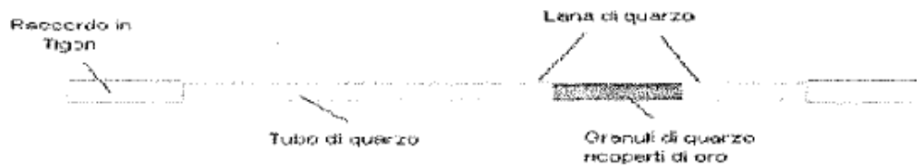
Fig.1 SCHEMA TRAPPOLA DI CAMPIONAMENTO
