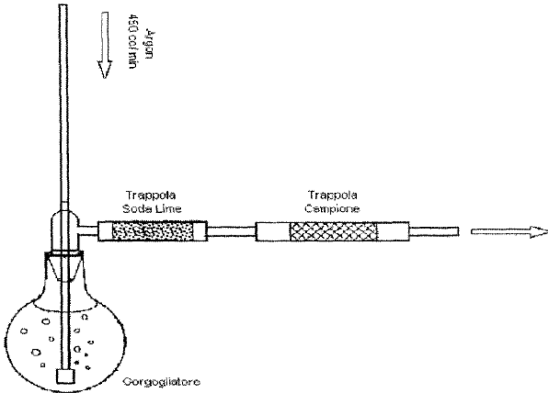
Figura 3 - Schema della tecnica Purge and Trap
