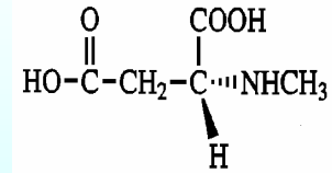
N-metil-D-Aspartato (NMDA)
