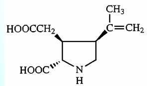
Kainato
