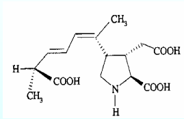
Acido domoico
