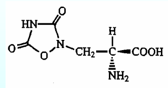
Quisqualato
