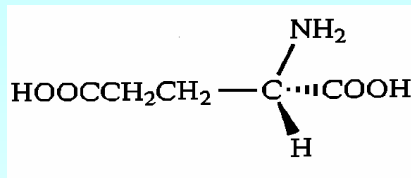
L-glutammato
