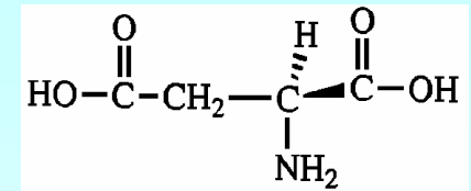
L- aspartato
